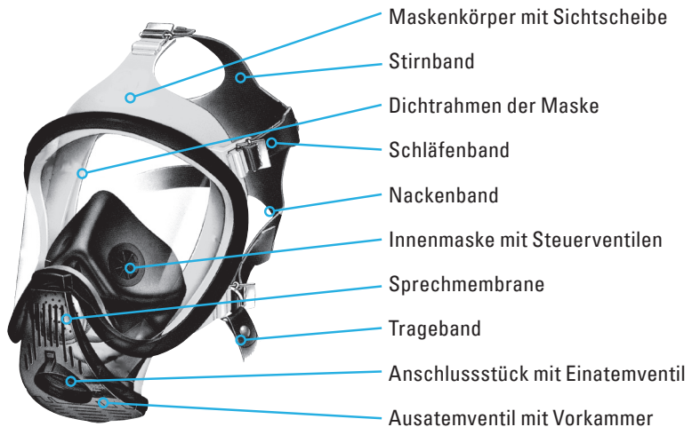
Abb. 2 Aufbau Atemanschluss
