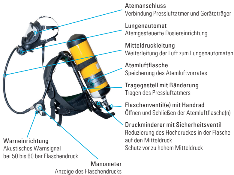
Abb. 5 Aufbau Pressluftatmer
